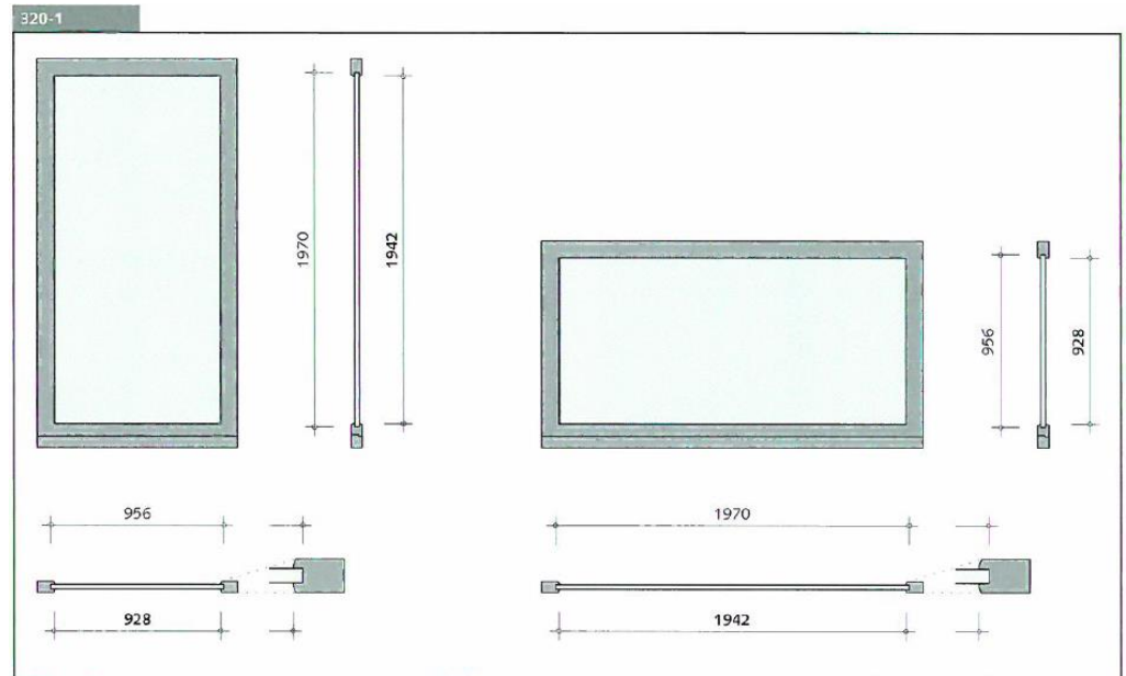
320-1 Maximale Glas-, Flügel- und Rahmen- Abmessungen (Angaben in mm)
