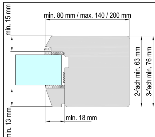
320-2 Minimale Abmessung des Rahmen- querschnitts (Angaben in mm)
