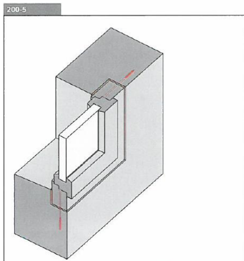
200-5 Einbau in abgestufte Unterkonstruktion, Befestigung zwischen Leibung
