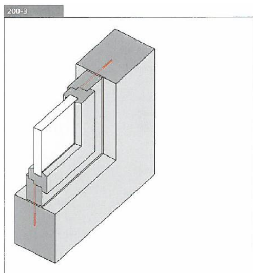
200-3 Einbau zwischen Leibung
