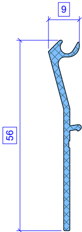
HS Abdichtblech horiz 56/9 oben Code: S1-AD 009-56 Lieferant: Koch AG 85.248.168 eloxiert
