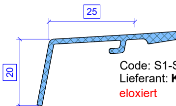
Code: S1-ST- 065-10 (eloxiert) Lieferant: Koch AG 88.045.06 eloxiert
