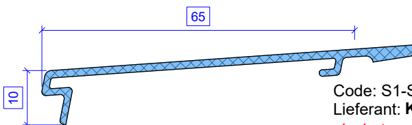
Code: S1-ST- 045-10 (eloxiert) Lieferant: Koch AG 88.045.04 eloxiert
