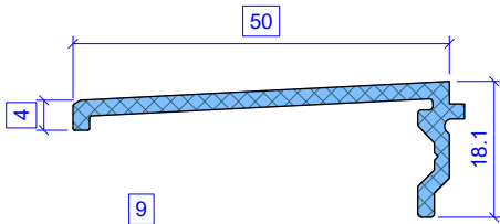
HS Abdichtblech horiz 56/9 oben Code: S1-AD 009-56 Lieferant: Koch AG 85.248.168 eloxiert
