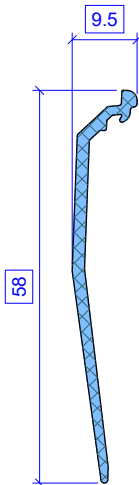
HS Abdichtblech horiz. 58/8 unten Code: S1-AD 008-58 Lieferant: Koch AG 85.981.268 eloxiert
