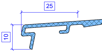
Code: S1-ST- 025-10 (eloxiert) Lieferant: Koch AG 88.045.02 eloxiert
