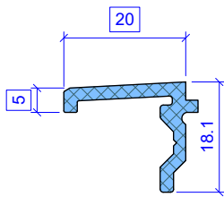
HS Steckteil B20 eloxiert Code: S1-ST 020-05 Lieferant: Koch AG 85.247.100 eloxiert
